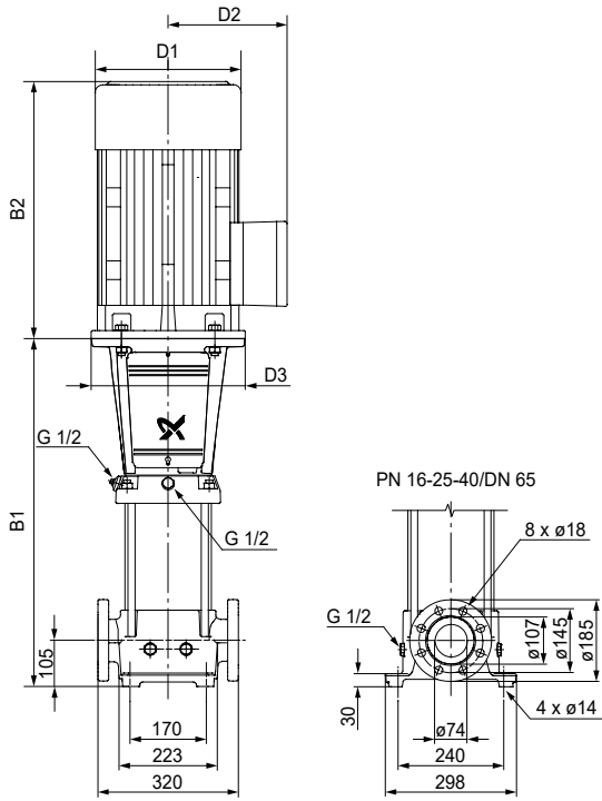
CR 32
