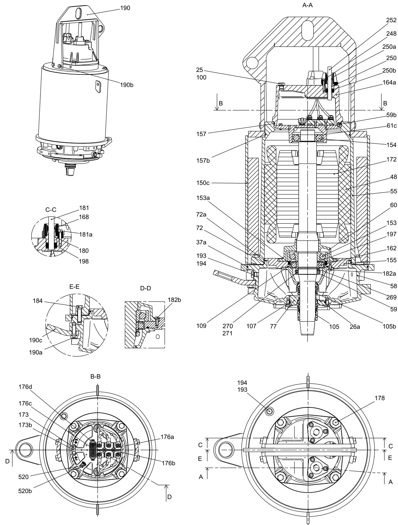
Рис. 24 Стандартный электродвигатель с охлаждающим кожухом
