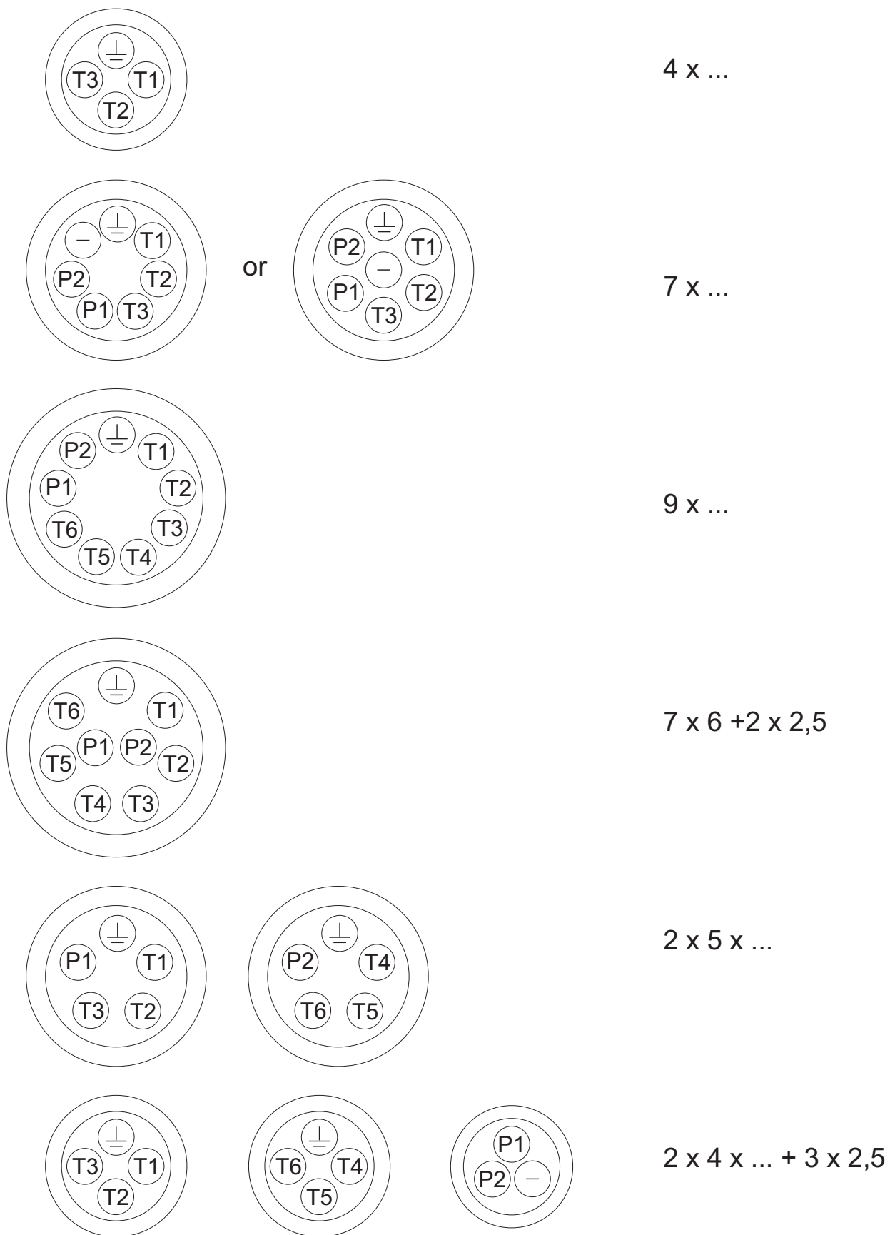
Рис. 40 Концы кабеля (со стороны свободного конца)
