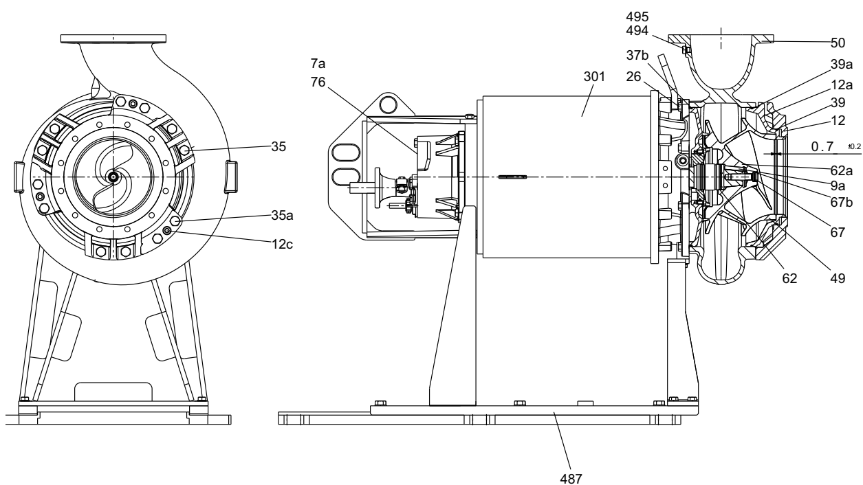
Рис. 37 Сухая установка насоса в горизонтальном положении, тип монтажа Н (2)
