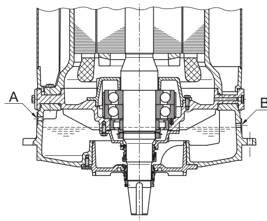
Рис. 9 Надлежащий уровень масла в насосе в вертикальном положении
