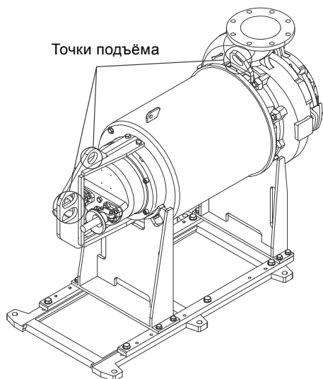
Рис. 2 Точки подъёма для типа монтажа Н
