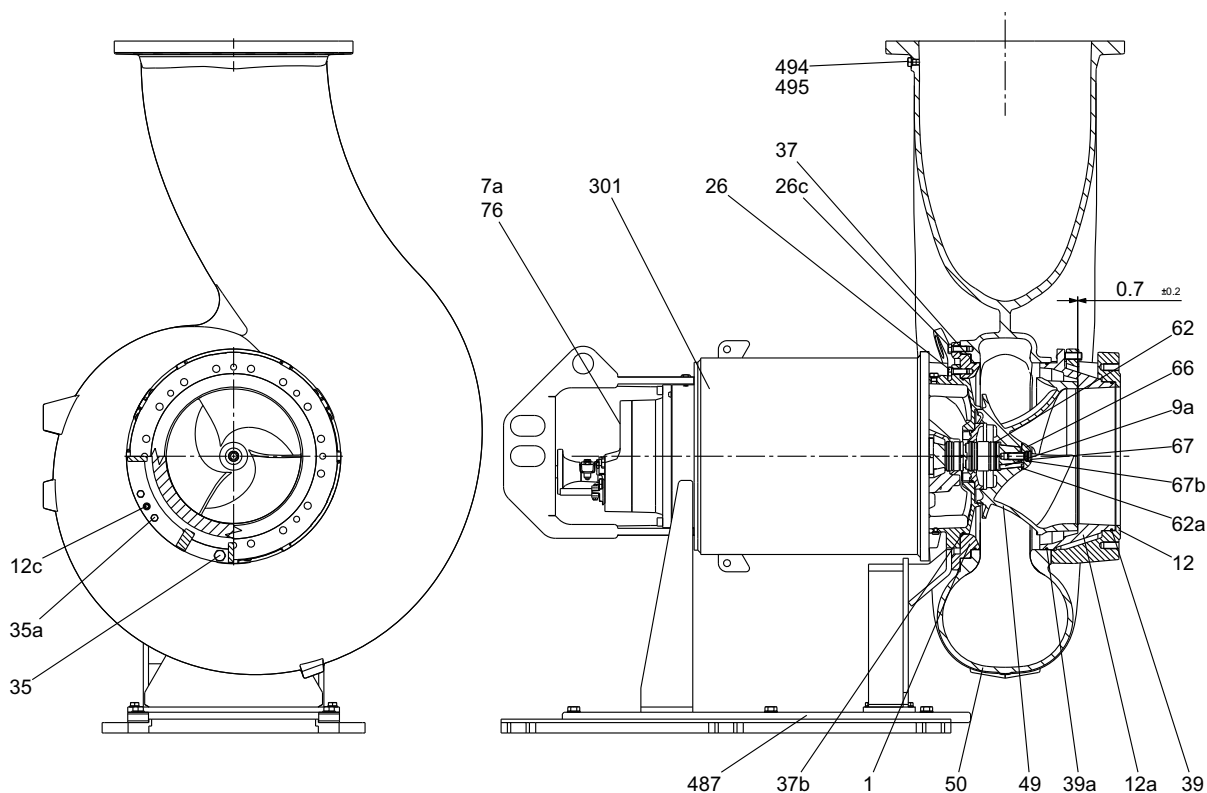
Рис. 36 Сухая установка насоса в горизонтальном положении, тип монтажа Н (1)
