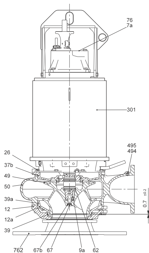
Рис. 35 Установка насоса, тип монтажа D (2)
