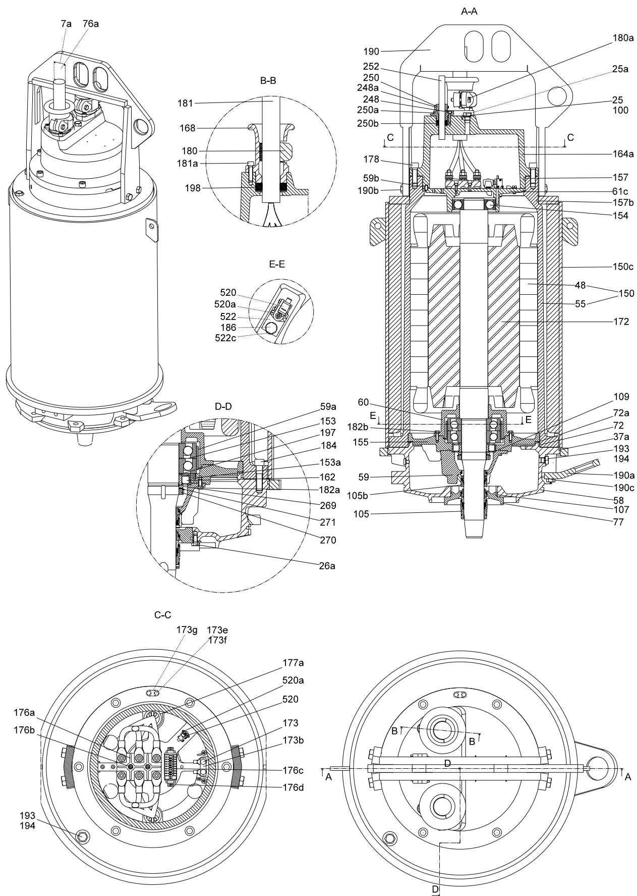
Рис. 30 Взрывозащищённый электродвигатель с охлаждающим кожухом
