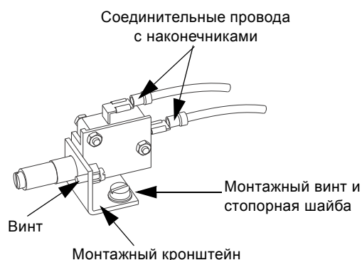
Рис. 14 Реле влажности
