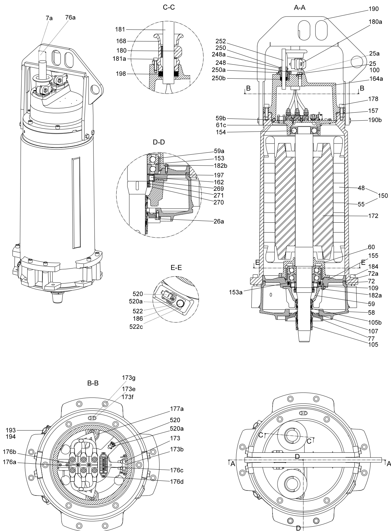
Рис. 29 Взрывозащищённый электродвигатель без охлаждающего кожуха
