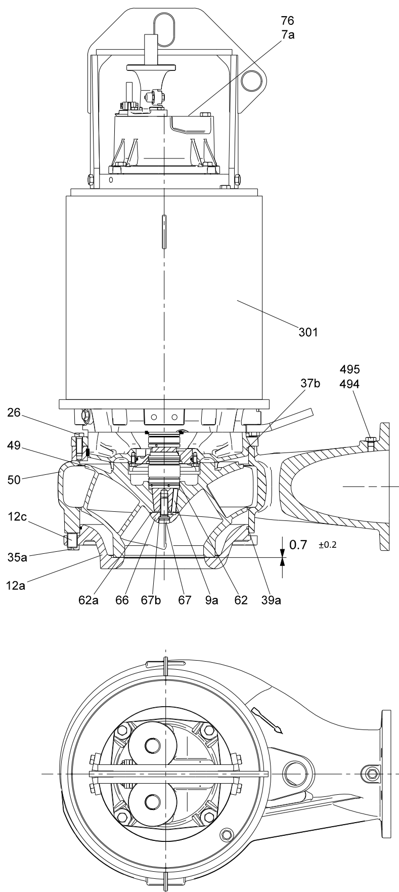
Рис. 31 Установка насоса в погружном положении с охлаждающим кожухом
