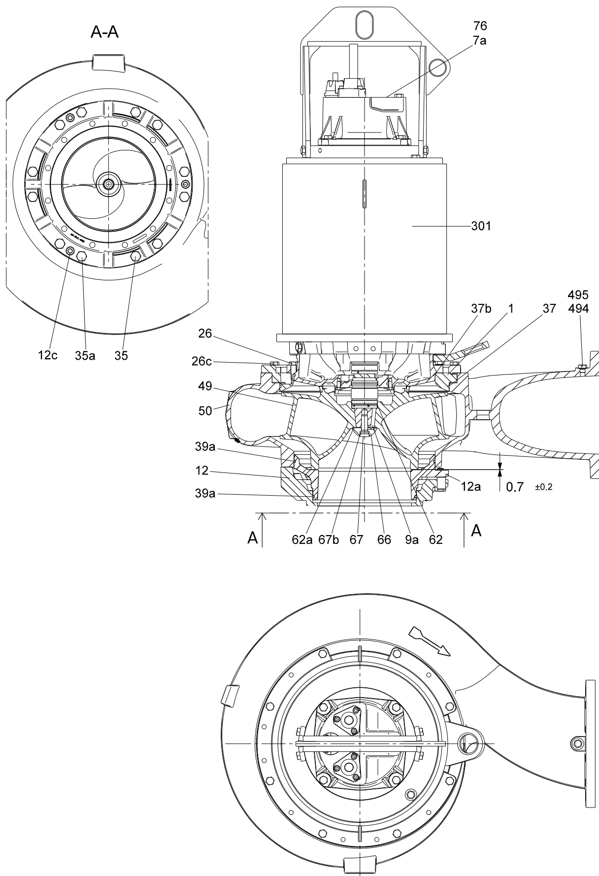
Рис. 32 Сухая установка насоса с охлаждающим кожухом
