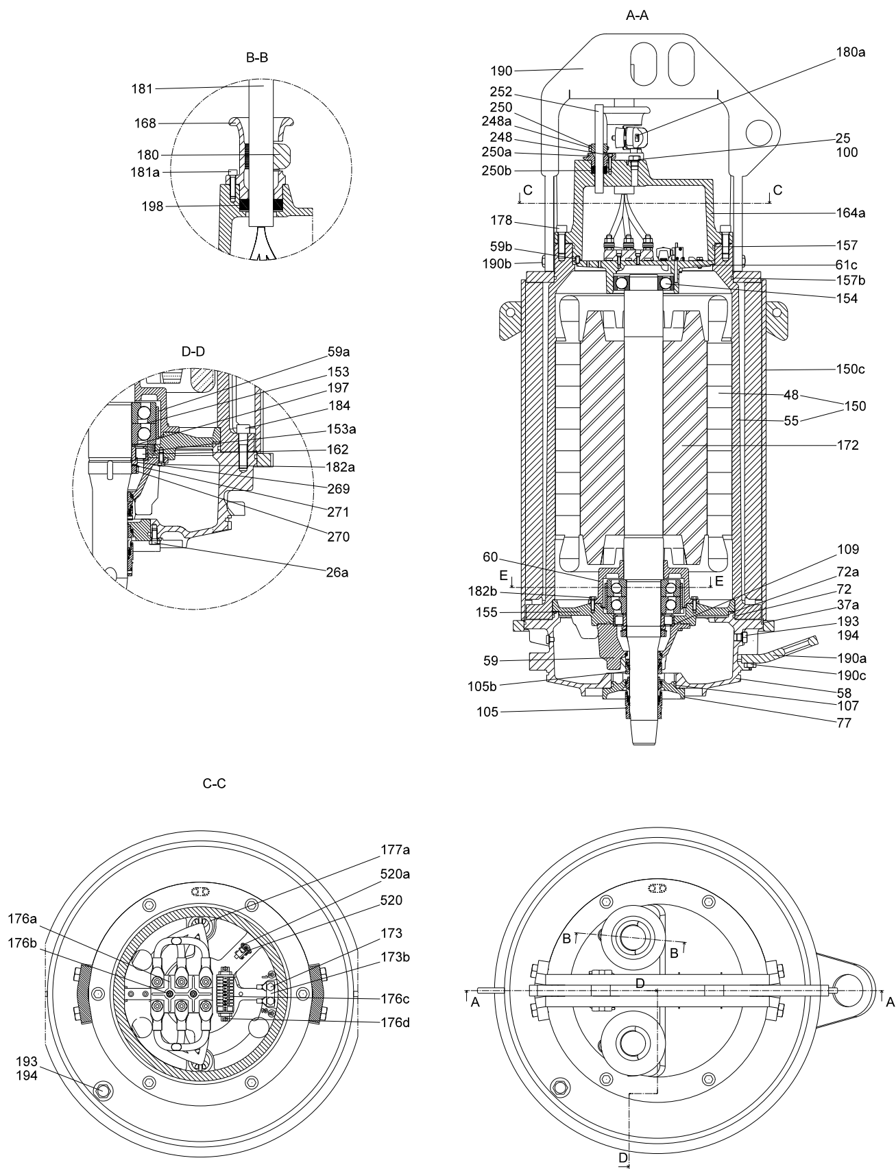
Рис. 28 Стандартный электродвигатель с охлаждающим кожухом
