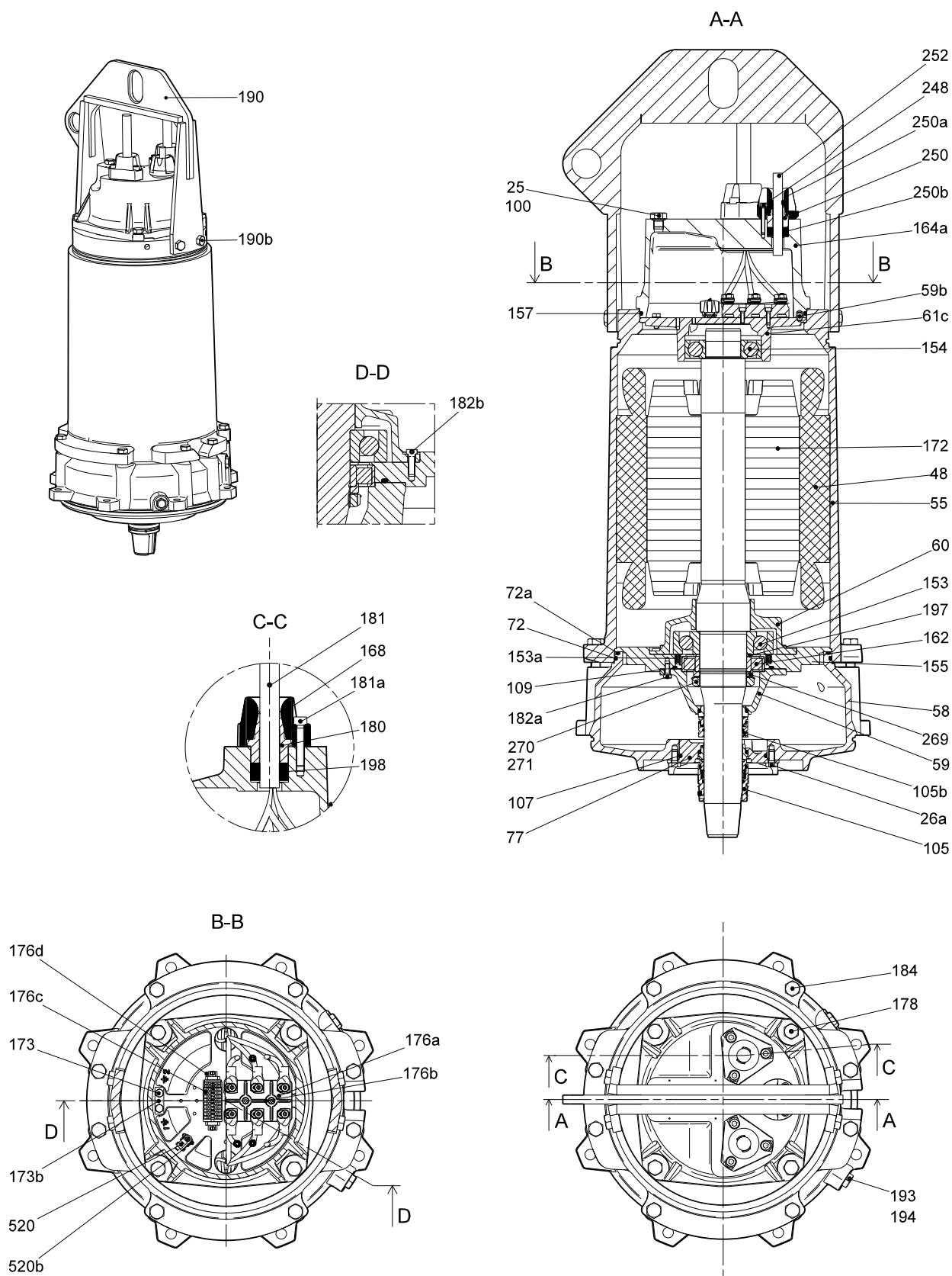
Рис. 23 Стандартный электродвигатель без охлаждающего кожуха
