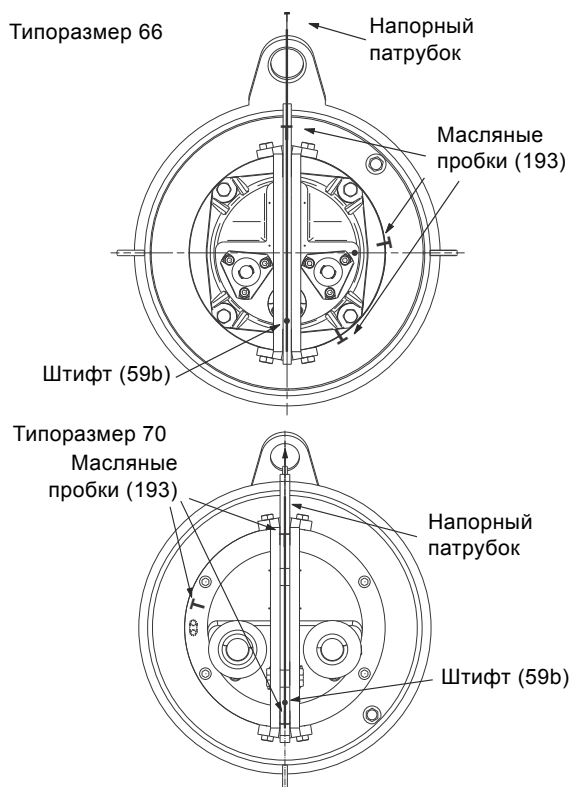
Рис. 21 Положение подъемной скобы, типы монтажа С, D и H
