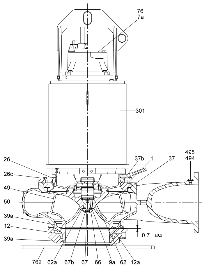
Рис. 34 Установка насоса, тип монтажа D (1)
