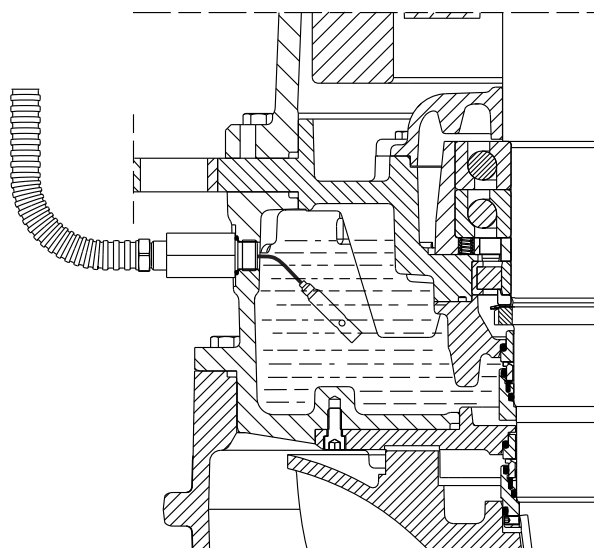
Рис. 16 Внешний датчик воды в масле (WIO)
