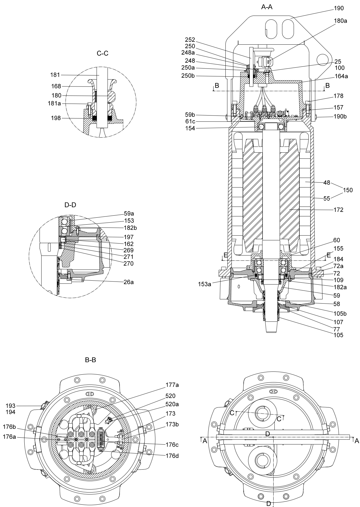
Рис. 27 Стандартный электродвигатель без охлаждающего кожуха
