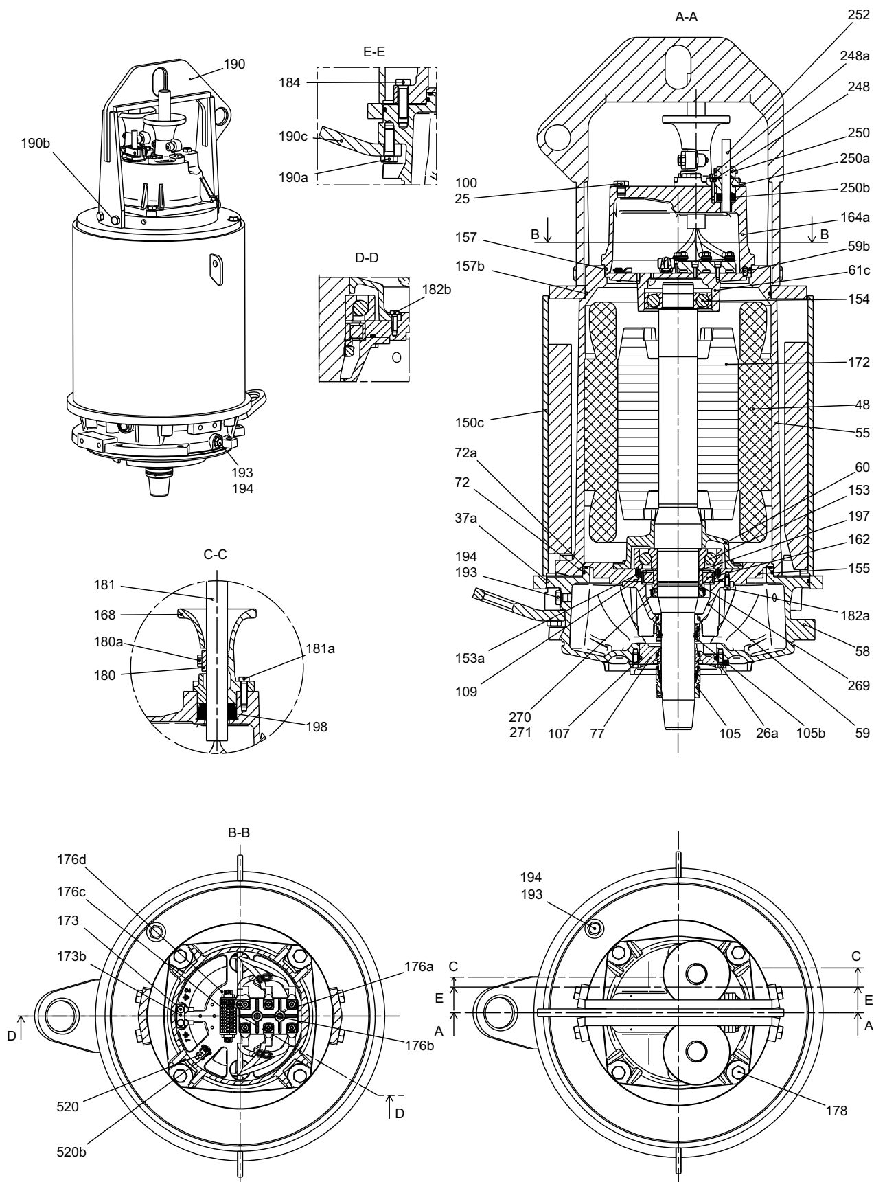
Рис. 26 Взрывозащищённый электродвигатель с охлаждающим кожухом
