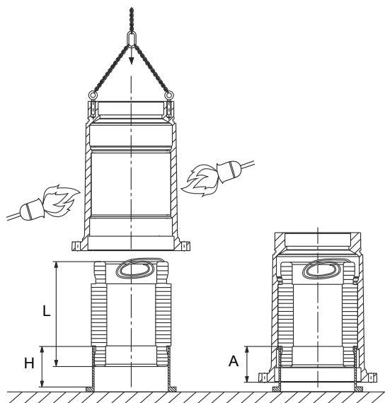
Рис. 19 Установка статора
