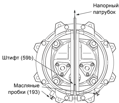
Рис. 20 Положение подъемной скобы, тип монтажа S
