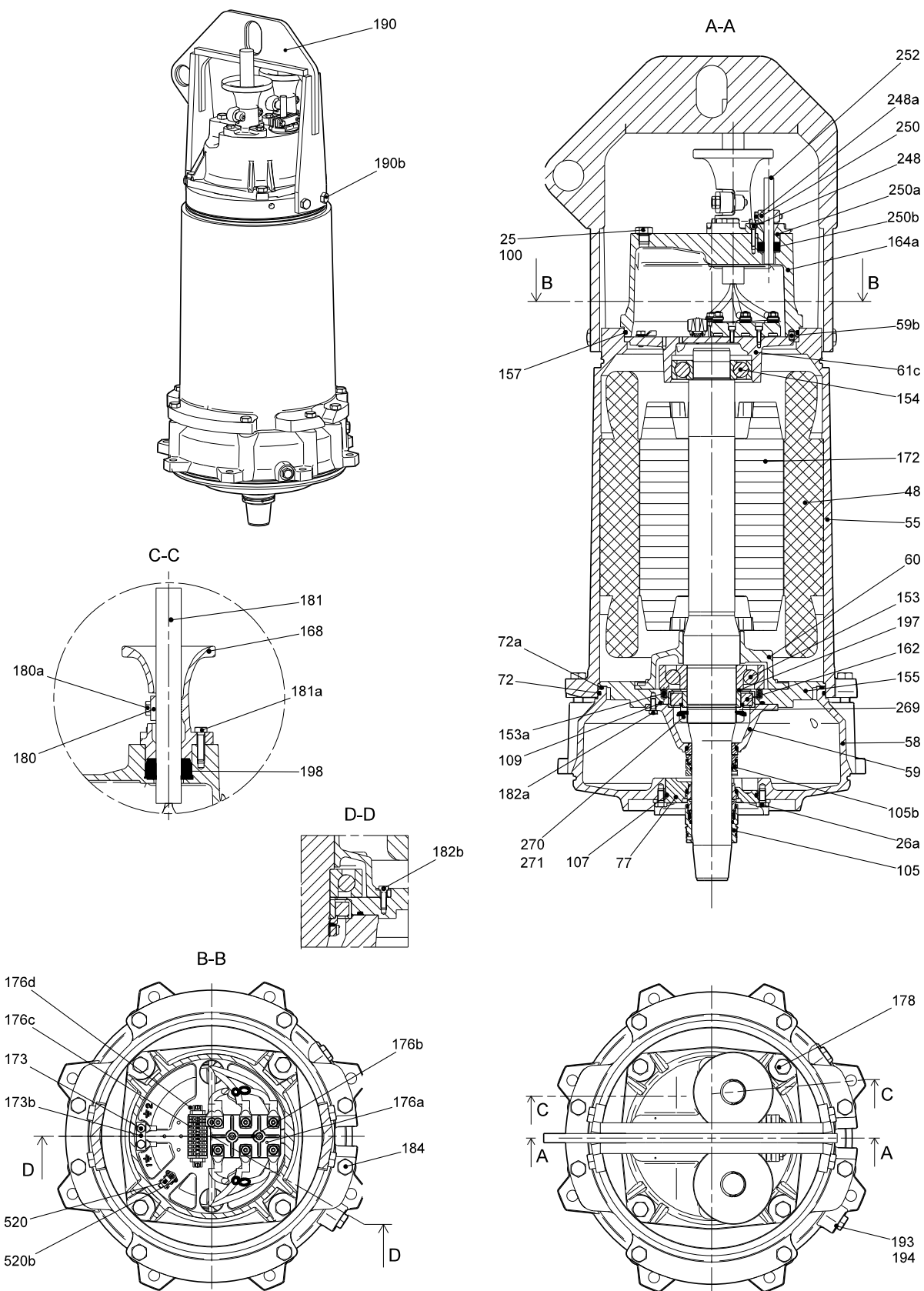
Рис. 25 Взрывозащищённый электродвигатель без охлаждающего кожуха
