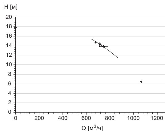
Рис. 21 Измеренные значения для расхода и напора.
