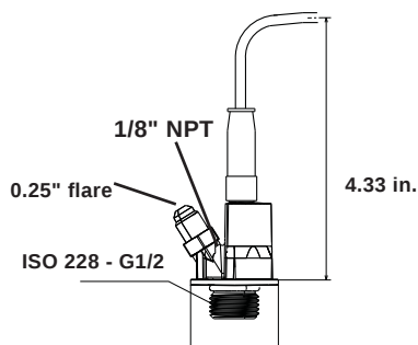
Fig. 60 Dimensions DPI/DPI+T
