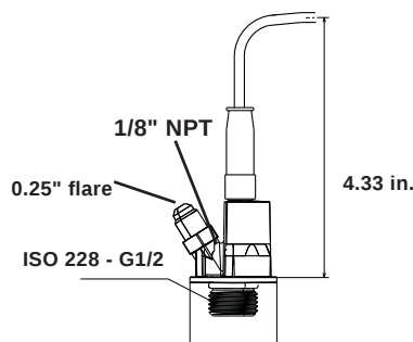
Fig. 56 Dimensions DPI/DPI+T
