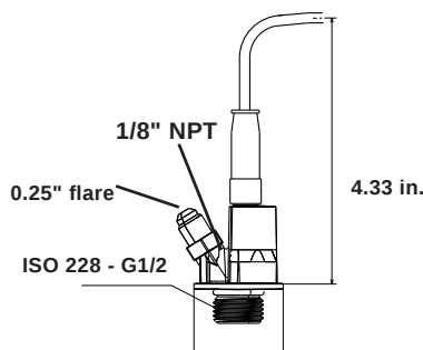
Fig. 52 Dimensions DPI/DPI+T
