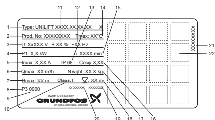
Ejemplo de placa de características
