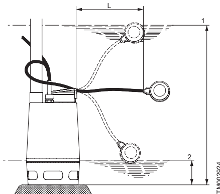
Niveles de arranque y parada
