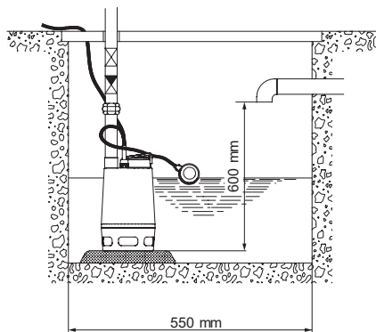
Colocación de la bomba sobre una placa
