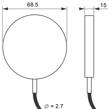
Fig. 3 Dimensions
